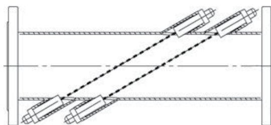
Прямая труба с многочуевым зондированием
