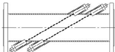
Прямая труба с многоручевым зондированием
