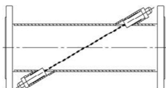
Прямая труба с одноручевым зондированием
